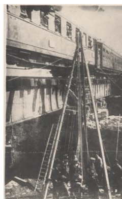
Prace porządkowe przy moście w Szczepanowicach pod Opolem, wysadzonym przez Grupę Destrukcyjną „Wawelberga” w nocy z 2 na 3 maja 1921 roku.
